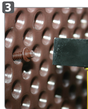
Frappez à l'aide d'un marteau
