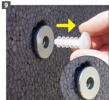
Une fois la résine durcie, retirez le bouchon de protection.
