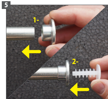
Anticipez en enfonçant la rondelle d'appui et le bouchon de protection dans le taraudage.
