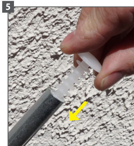
5 Anticipez en enfonceant légèrement le bouchon de protection dans le taraudage.
