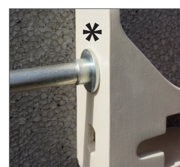
La rondelle d'appui est en place derrière le support pour éviter l'écrasement.
