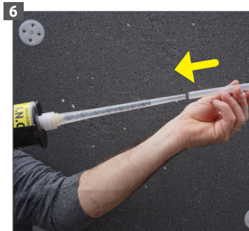
Placez la rallonge sur l'embout mélangeur et faites monter la résine jusqu'au bout.
