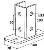
Pied profil acier lourd - schéma technique
