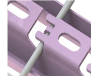
Equerre universelle LWU - pattes rabattables
