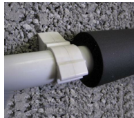
TUB-RING - vue en situation avec isolant
