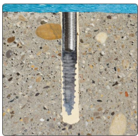
Douille Inox A4 à la résine - vue en coupe
