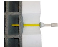
Arrêt de volet auto ISO - vue en coupe
