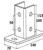
Pied profil acier lourd - schéma technique
