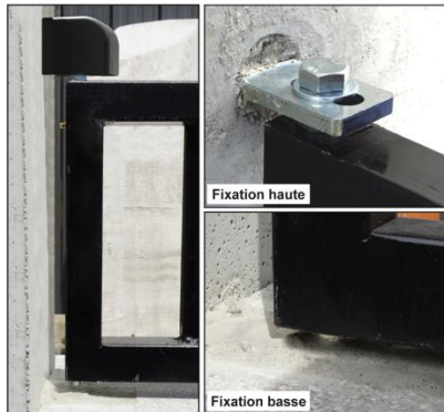
Pivot de portail à sceller pour portail acier avec seuil
