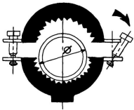
Collier 2 vis isolé isolant épais - schéma
