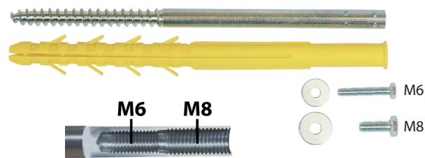
Vis taraudée M6 et M8
