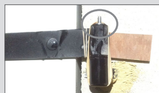
9 Mettre l'élastique pour maintenir le gond pendant le temps de séchage de la résine.
