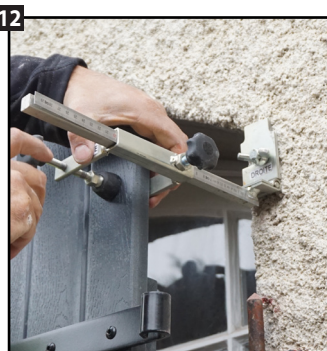
Ajuster la longueur selon l'épaisseur de l'isolant. Répéter l'opération de l'autre côté du volet.
