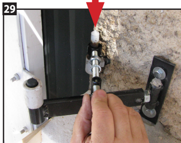
29 Positionner la pièce de raccordement entre l'ancien et le nouveau gond par dessus.
