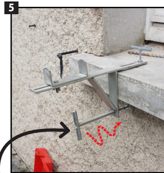
Serrer la pièce contre le crépi pour faire contrepoids.
