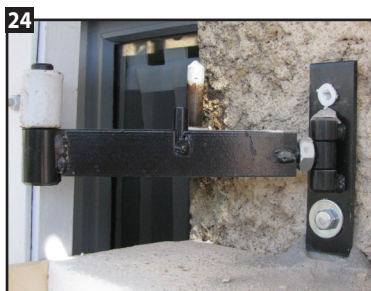
24 Mettre en place la cheville blanche à travers la platine.
