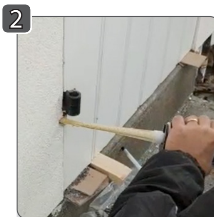
Injection de la résine dans le bloc isolant
