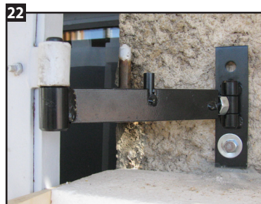
22 Après cette vérification, bloquer à fond.
