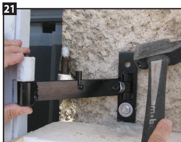
21 Si besoin, grâce au trou plus large, positionner parfaitement le gond en tapotant.
