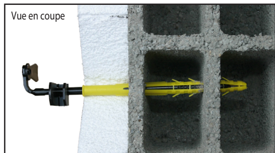
Dans le parpaing, expansion sur les deux alvéoles.
