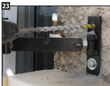
23 Percer Ø10 le trou supérieur à travers la platine.
