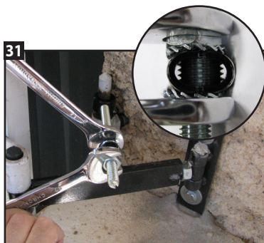
31 Blocage des 2 écrous en même temps pour garantir le bon maintien de l'écartement jusqu'à l'ovalisation de la pièce ronde.
