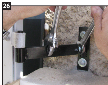
26 Si besoin, on peut redresser le gond en dévissant l'écrou zingué (clé de 17) en faisant bouger le fer plat à l'aide d'une clé à molette.
